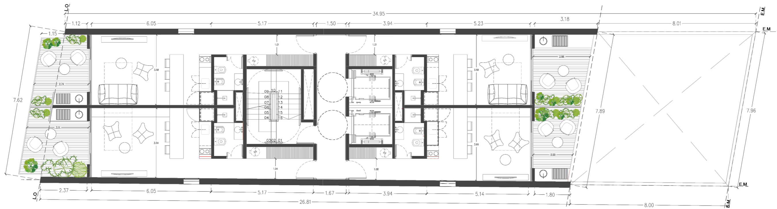
PLANTA TIPO 1° - 9°
